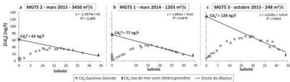
Fig. 2. Distribution des concentrations en Cd_d dans le gradient de salinité pour les trois missions MGTS 1 à 3. Les Cd_d^0 sont déterminées à l'aide des régressions linéaires représentant la dilution des eaux estuariennes par les eaux marines.
