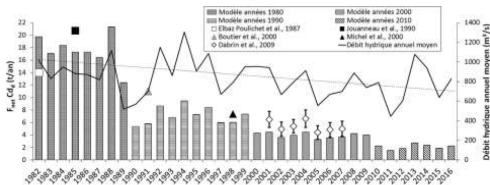
Fig. 7. Les barres grisées et hachurées donnent les variations interannuelles et inter-décennales des flux nets de Cd_d en tonne/an. La variation interannuelle des flux hydriques en m^3/s est également reportée. Les figurés blancs, noirs et gris correspondent aux valeurs des flux nets publiés antérieurement.
