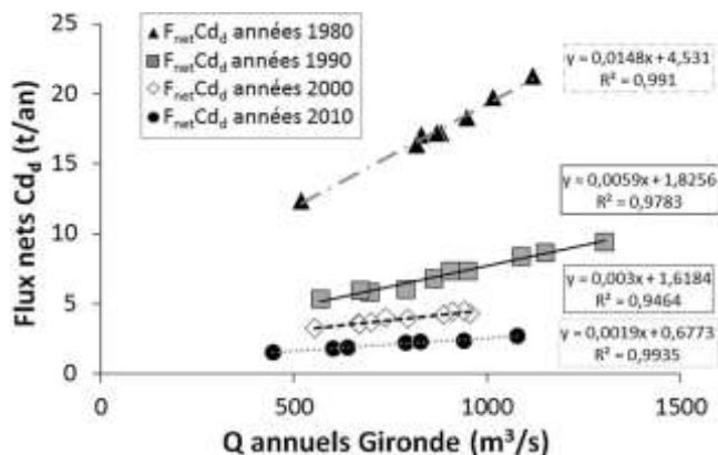
Fig. 8. Diagramme montrant les quatre régressions linéaires servant d'abaques pour l'estimation des flux nets annuels de cadmium dissous (Cd d ) exportés par la Gironde pour les quatre dernières décades.
