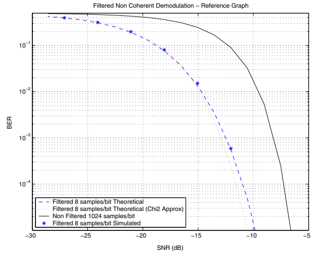
Fig. 5 REFERENCE BER
