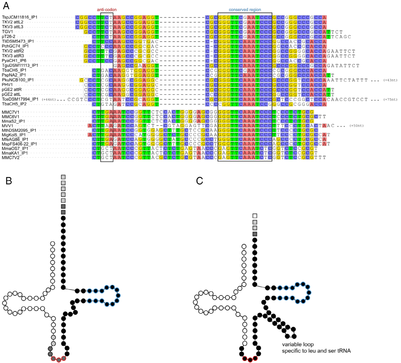
Fig. 6. att site variability.
