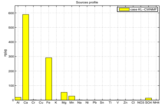
Fig. 5. KL-CWNMF: Steel slag profile
