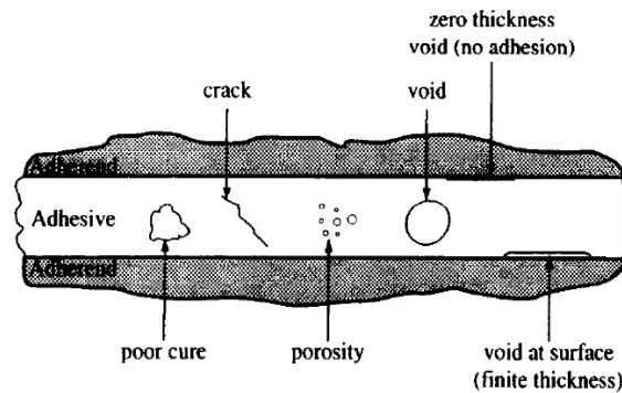
Figure 1 : Défauts dans un assemblage collé [7]
