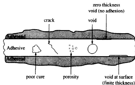
Figure 1 : Défauts dans un assemblage collé [7]
