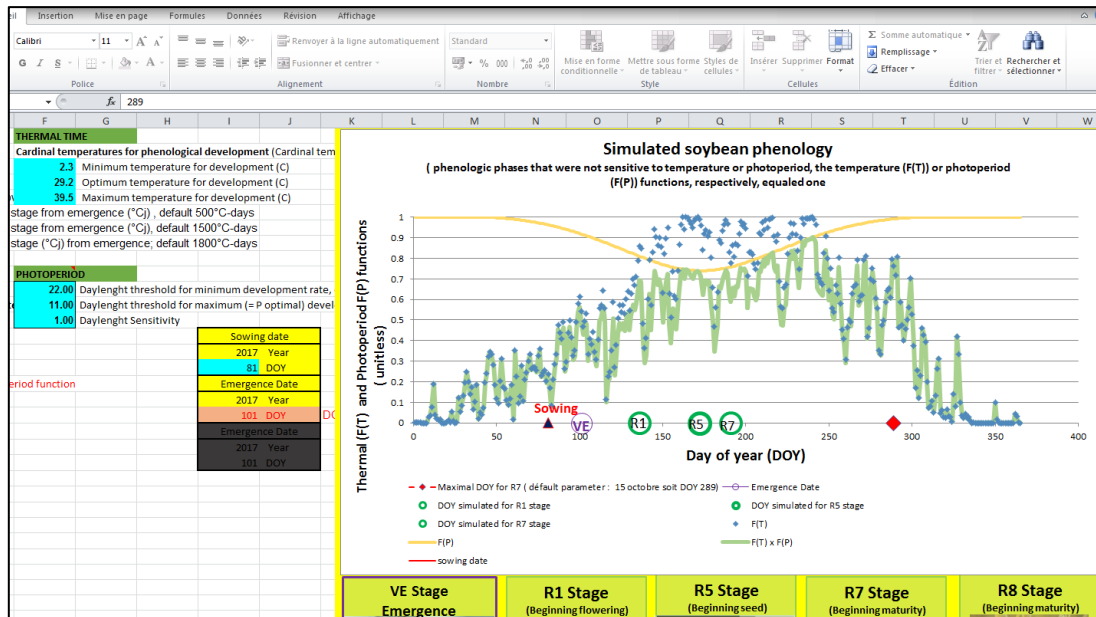
Figure 5 : Impression écran du modèle Phenology Simple et d'un graphique permettant de visualiser les fonctions thermique (f(T) en bleu), photopériodique (f(P) en jaune), et la combinaison des deux (f(T) x f(P) en vert) au cours du temps. Ces fonctions (valeurs comprises entre 0 et 1) permettent le calcul du temps photothermique journalier : (T_{opt} - T_{min}) \times f(T) \times f(P) , avec T_{opt} et T_{min} pour températures optimale et minimale, respectivement. Lorsque la fonction thermique - ou photopériodique - est égale à 1, les conditions thermiques - ou photopériodiques - sont optimales pour le développement. En revanche, l'accumulation du temps photothermique par le soja est diminuée par ces fonctions lorsque leurs valeurs sont inférieures à 1 ; il en résultera un allongement en jours de la durée de la phase phénologique pour satisfaire l'exigence photothermique de la variété. Les jours d'apparition des stades phénologiques clés pour la situation de production simulée sont représentés par des cercles.
