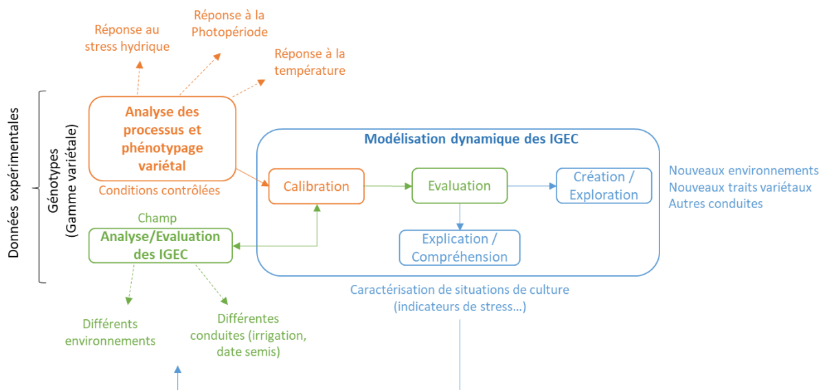
Figure 1 : Schéma général de la démarche d'analyse et de modélisation des interactions génotype-environnement-conduite (IGEC). Cette démarche peut s'appliquer à différents processus écophysologiques mais sera utilisée ici pour étudier la phénologie. Le phénotypage des variétés en conditions contrôlées et au champ (données expérimentales) sert à calibrer puis évaluer des modèles de culture plus ou moins complexes. Dans cette étude, les données issues des expérimentations en conditions contrôlées, les plus précises, serviront de base de calibration ; l'évaluation du modèle sera réalisée à l'aide d'un jeu de données « champ ». Le modèle ainsi calibré et évalué servira à donner des clés de lecture des données expérimentales et permettra l'exploration de nouvelles conditions culturales.
