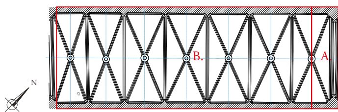
Figure 72 a : Principe de renfort des couchis mis en place entre les gorges des ogives et des arcs doubleaux – éch. : 1/50 : - Doubleau de la croisée du transept (D_8) et branches d'ogives de la travée 9 du vaisseau central. - Doubleaux et branches d'ogives du vaisseau central.
