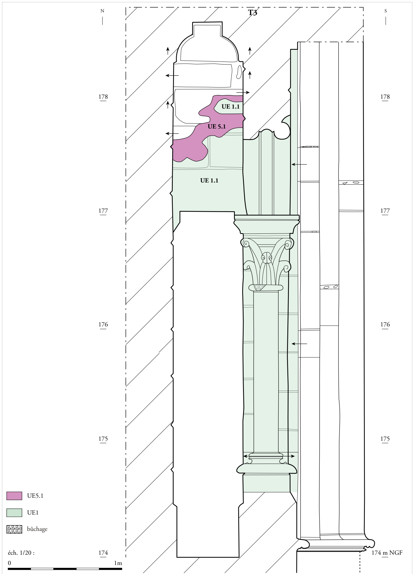
Figure 117 : Travée 3 nord : coupe nord-sud de la galerie du triforium - éch. : 1/20.
