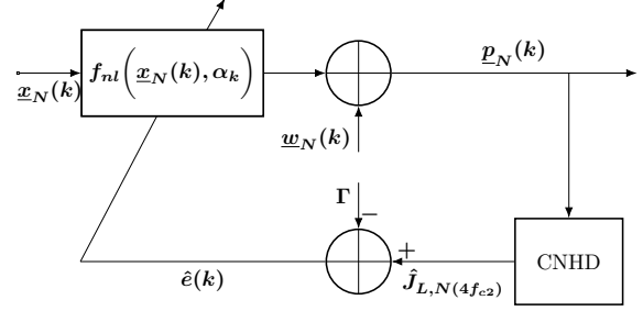
FIGURE 1 – Boucle de rétroaction de gain basée sur une détection cyclostationnaire d'harmoniques non linéaires
