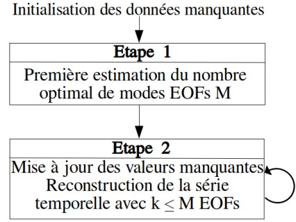
FIGURE 1 – Diagramme la méthode EM-EOF en deux phases. Les données manquantes sont d'abord initialisées. La phase 1 effectue une première estimation du nombre optimal de modes EOF M qui minimise l'erreur de reconstruction. La phase 2 est un affinage itératif des valeurs manquantes pour reconstruire la série temporelle avec un nombre k d'EOFs.
