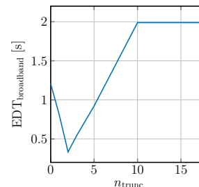
(d) EDT.
