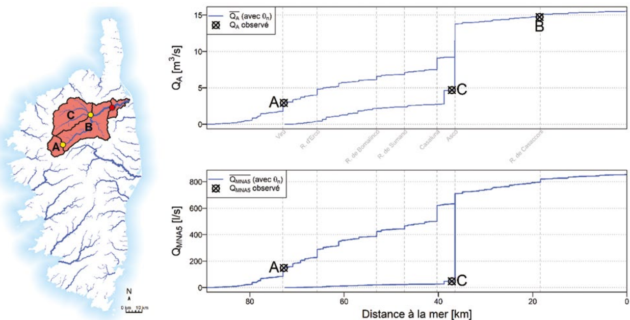
Figure 6 : Évolution du Q_A et du Q_{MINAS} le long du Golo et de son principal affluent, l'Asco. Les valeurs de références calculées aux stations hydrométriques du bassin versant sont également représentées.
