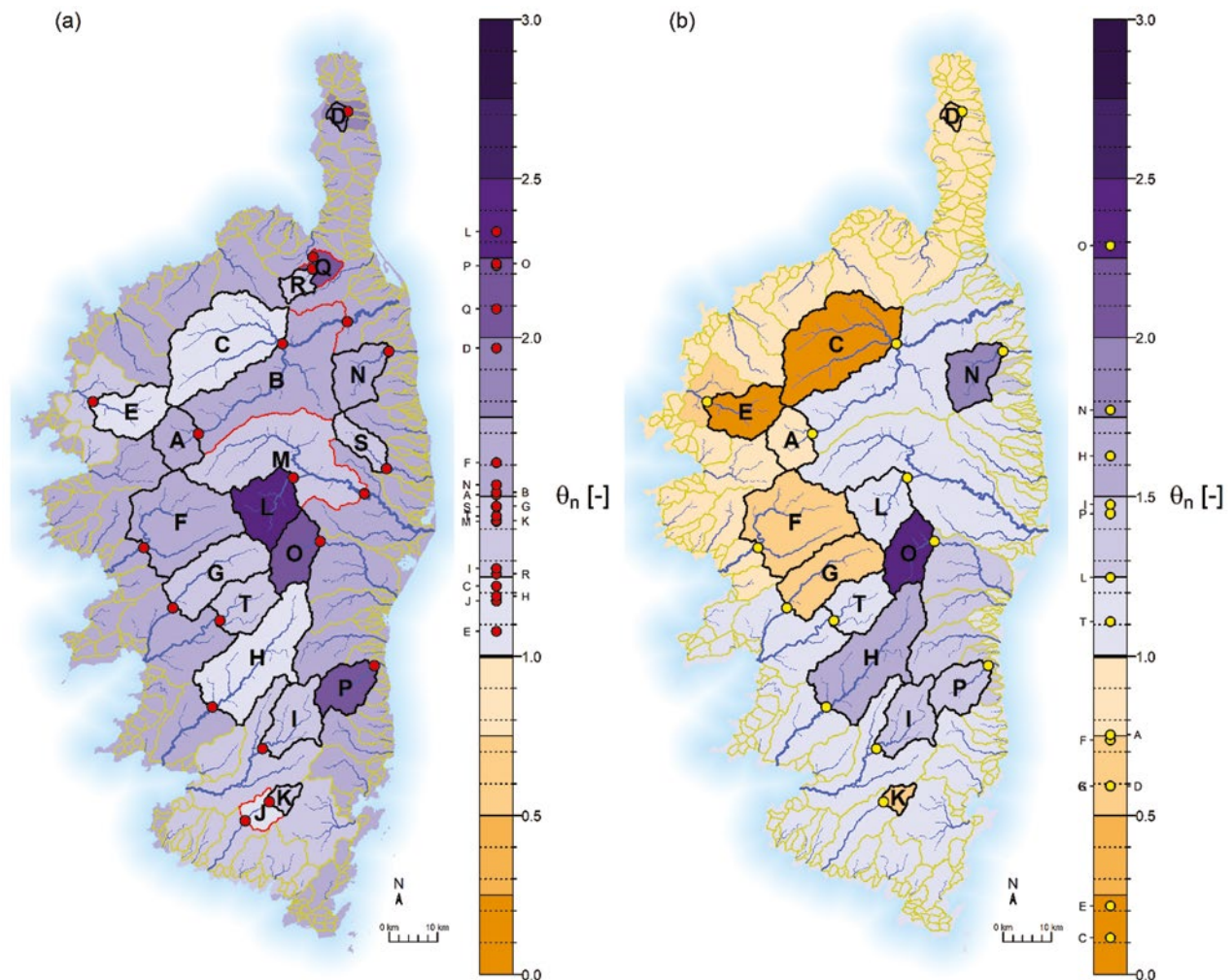
Figure 4 : Valeurs de facteurs correctifs ( \theta_n ) pour la cartographie de Q_A (a) et de Q_{MNA5} (b), calculés pour chaque maille du MNT à partir des bassins versants étudiés (bassins « amont » en noir, bassins « aval » en rouge). Les contours des bassins versants non-jaugés drainant plus de 2 km 2 sont représentés en jaune foncé.
