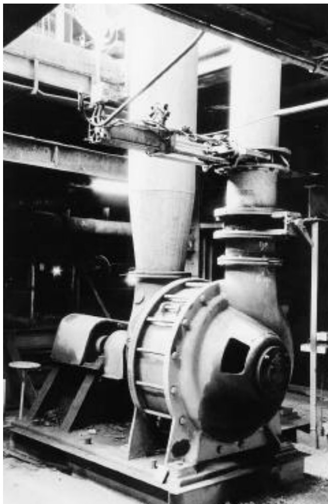
2) Turbine dite « soufflante » alimentant les bacs P. I. C. (cl. F. Pillet © Ecomusée, 1999 ; Inventaire général, ADAGP, 1999)
