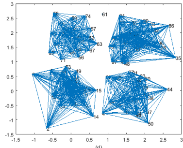
(d) Completion of R^{\varepsilon^*} with zeros
