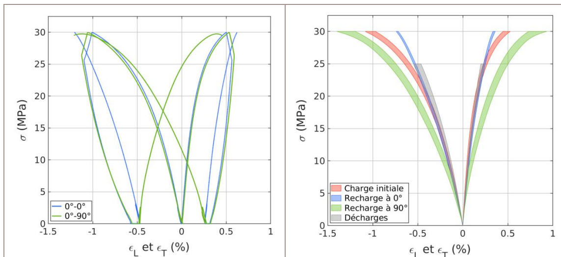
Figure 11 : Exemple de courbes contrainte-déformations d'essais de compression 0°-0° (en bleu) et 0°-90° (en vert).
