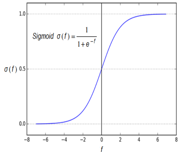
Fig. 4. Sigmoid Function
