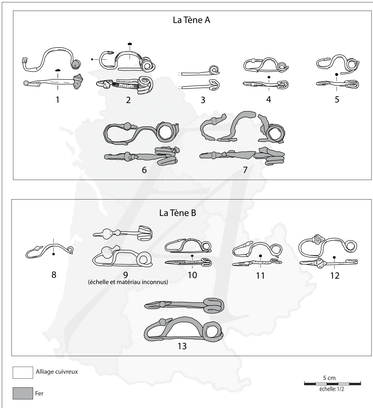
Fig. 3. 1. Les Châteliers à Paizay-Naudouin-Embourie, Charente (Gomez de Soto et al. 2007) ; 2. La Calévie à Mayrals, Dordogne (Chevillot et al. 1977) ; 3. Place Malu à Saint-Martin-des-Champs, Cher (Milcent 2004, pl. 27) ; 4. Tombe 48, En Pétoleyres à Saint-Sulpice, Vaud, Suisse (Kaenel 1990, pl. 42) ; 5 à 7. Tombe 44, En Pétoleyres à Saint-Sulpice, Vaud, Suisse (Kaenel 1990, pl. 40) ; 8. La Grange à Surgères, Charente-Maritime (Giraud & Gomez de Soto 1996) ; 9. Provenance inconnue (Baray et al. 2007) ; 10 à 12. Belmont-sur-Yverdon, Vaud, Suisse (Kaenel 1990, pl. 7) ; 13. Longchamp à Bouqueval, Val-d'Oise (d'après Guadagin 1984, in : Marion 2004, fig. 250).
