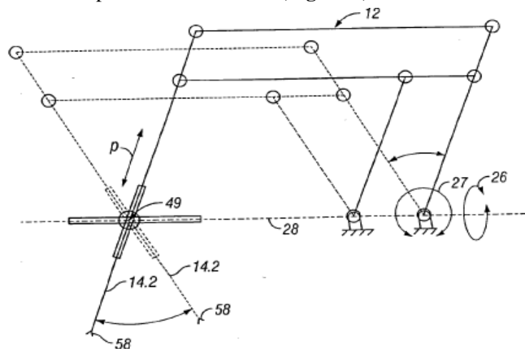
Figure 2 : RCM issu du brevet US20070038214
