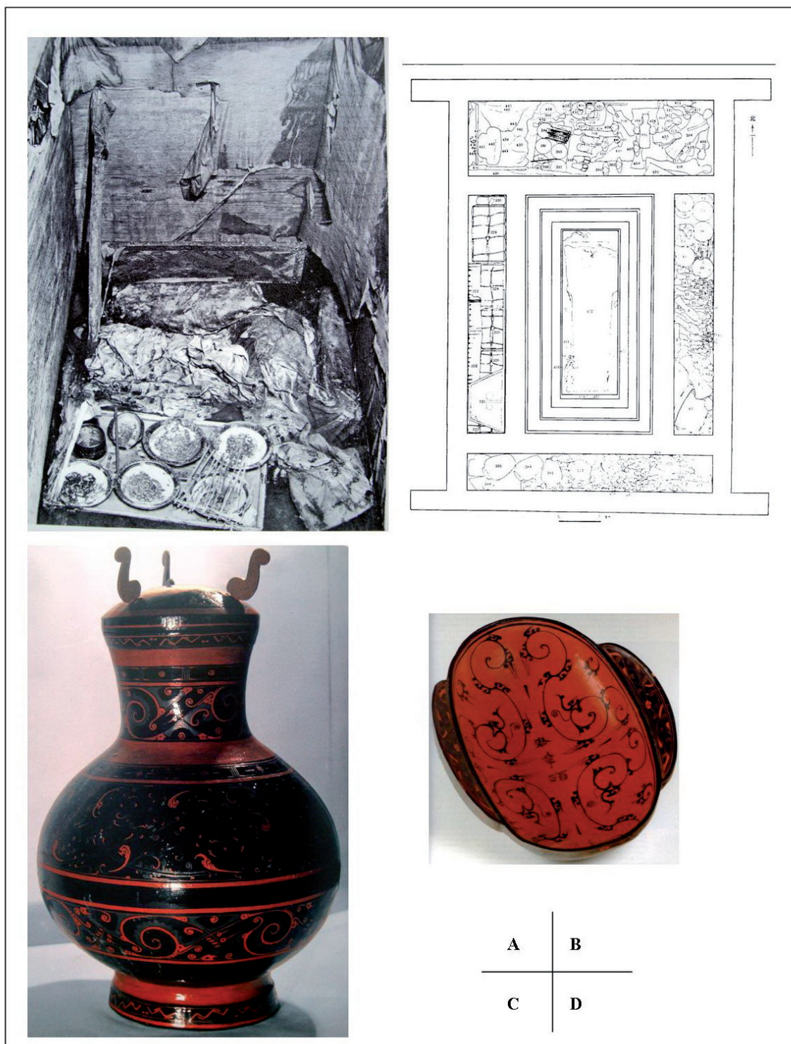
Fig. 8 - Tombe de la marquise de Dai à Mawangdui (Changsha, Hunan). Dynastie des Han occidentaux (vers 165 avant J.-C.) : A. repas funéraire, B. plan de la tombe, C. vase à vin en laque, D. coupe à oreilles pour le vin en laque (d'après Pirazzoli-t'Serstevens 1992 : 102, 129).
