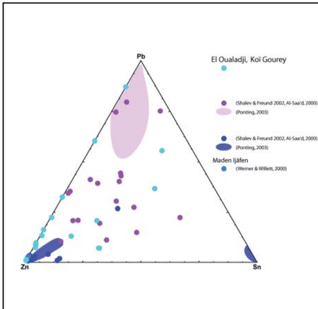
Fig. 9. Diagramme ternaire montrant les teneurs relatives en zinc, étain et plomb pour différents objets en métal base cuivre : des objets provenant de deux tumulus du delta intérieur du Niger (Mali), des objets issus de différents sites du Proche-Orient musulman du XIe-XIIIe-XIIIe s. et les trois barres analysées du Ma'den Ijâfen. Pour les objets provenant de sites du Proche-Orient médiéval musulman, on a séparé les objets obtenus par martelage de ceux obtenus par fonte afin de mettre en évidence une association nette entre mise en forme du métal et nature de l'alliage. Graphique et PAO : B. Mille (C2RMF).
