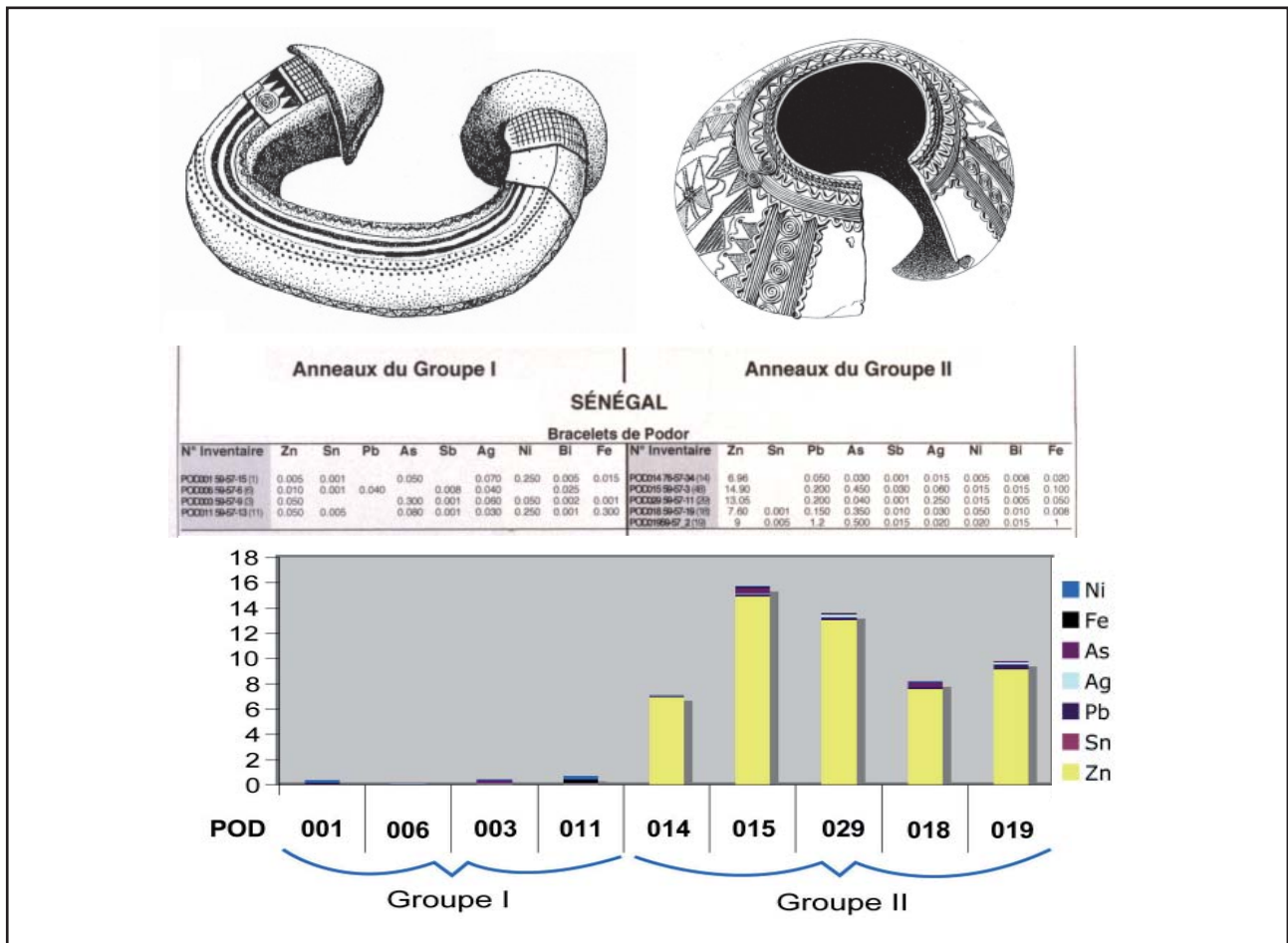
Fig. 3. Résultats des analyses élémentaires conduites sur des anneaux de la cache de Podor appartenant à deux séries typologiques distinctes. On observe une nette partition du métal entre les deux groupes : cuivre «rouge» pour les anneaux du Groupe I et laiton pour ceux du Groupe II.
