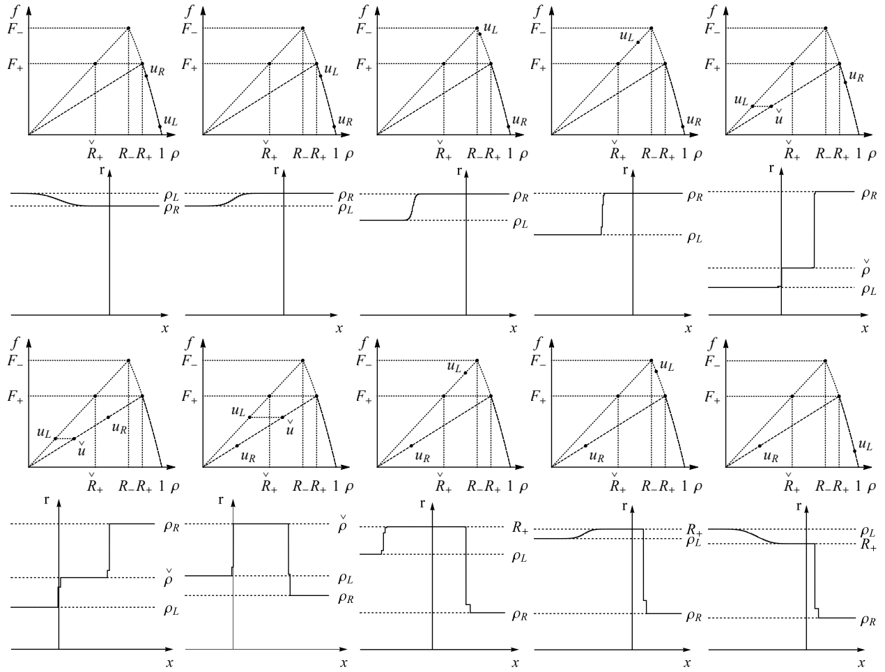
Fig. 2. Case V_+ < V_- < 1/2 .
