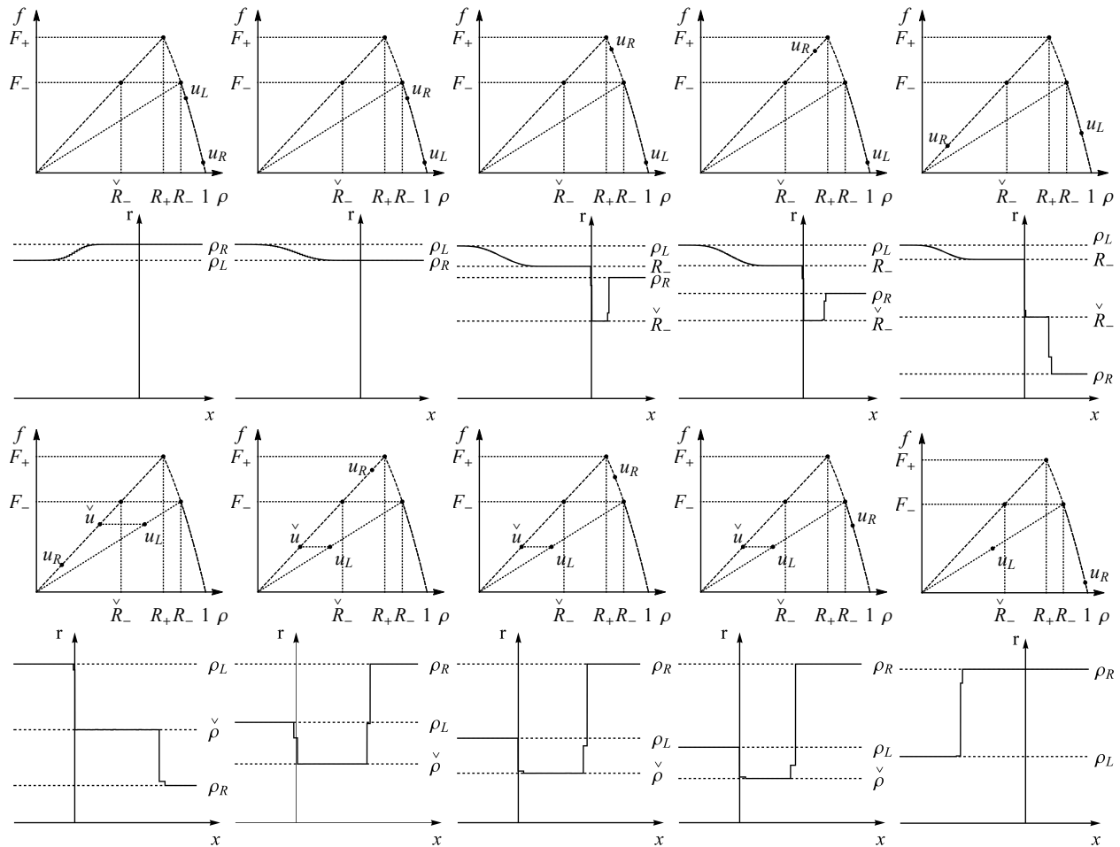
Fig. 1. Case V_- < V_+ < 1/2 .
