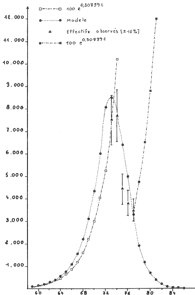
FIG. 1. — Evolution des effectifs de chats harets ( Felis catus L.) aux îles Kerguelen. Sont figurés, les effectifs observés (PASCAL, 1980), les résultats obtenus d'après le modèle mathématique développé par PASCAL (1977) et ceux obtenus par le modèle proposé par DERENNE (1976) ( 100 e^{0,30839 t} ). Les campagnes d'éradications ayant été interrompues en 1977, le modèle proposé par DERENNE redevient valable après cette date (toutes choses restant égale par ailleurs) et permet de prévoir une population de l'ordre de 12 000 félins en 1981.
