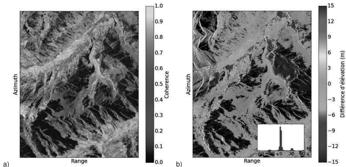
Figure 7 : (a) Cohérence interférométrique pour la paire TDX 2012/05/24; (b) Différence d'élévation entre les MNE TDX obtenus en utilisant comme référence le MNE SRTM ou un MNE Pléiades, d'après (Dehecq et al., 2016). L'encart montre l'histogramme des différences d'élévation. L'arrière-plan est l'image en amplitude TDX : les zones d'ombre apparaissent très sombres alors que les zones de recouvrement apparaissent très lumineuses. Les régions déconnectées du reste de l'image par les ombres/repliements (faible cohérence) présentent fréquemment des sauts de phase (en bleu et rouge sur l'image (b)).
