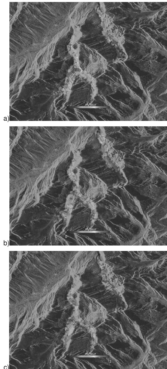
Figure 11 : Cartes de magnitude des déplacements \vec{V}_{SAR} estimés à partir des couples d'images Sentinel-1 ascendantes : asc (a) Couple 20-26/12/2017, (b) Couple 20/08-01/09/2017, (c) Couple 20/08-07/09/2017. Les résultats, en géométrie radar sont incrustés sur une image d'amplitude moyennée à partir des 4 images SAR ascendantes des couples correspondants.
