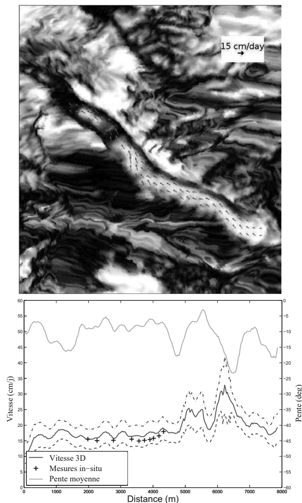
Figure 3 : Mesure D-InSAR du mouvement du glacier d'Argentière (ERS, 10-11 mars 1996) convertie en vitesse 3D sous l'hypothèse d'écoulement dans la direction de plus grande pente ; composantes horizontales superposées sur la cohérence ortho-rectifiée et profil longitudinal du module de la vitesse 3D comparé aux mesures in-situ et à la pente, d'après (Vasile, 2007).
