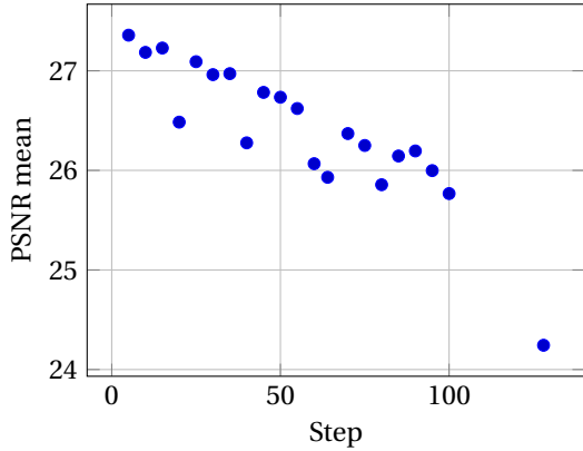
(b) PSNR
