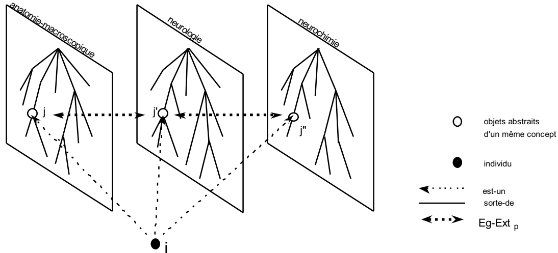
Figure 2 : Organisation de la base de connaissances par domaines
