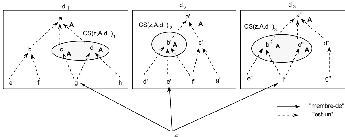
Figure 6 : Exemple de graphe d'héritage avec des conflits intra et inter-domaines
