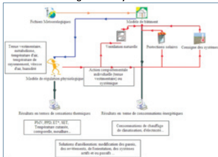
Figure 2: Exemple de plate-forme de simulations sur le logiciel TRNsys
