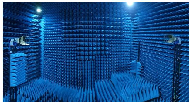
Figure 5. Chambre anéchoïque utilisée pour la mesure de gain du prototype
