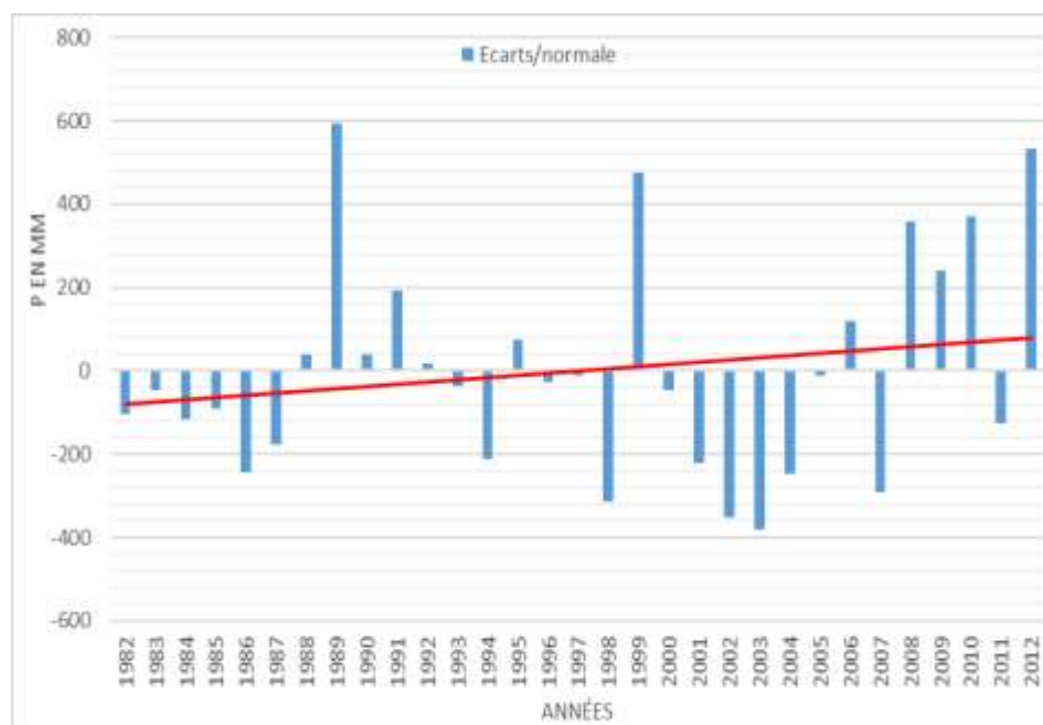
Figure 2 : La variabilité pluviométrique à la station du Cap-Skirring (1982-2012)
