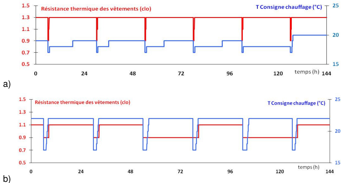
Figure 5 : Tenue vestimentaire (rouge) et température de consigne (bleu) pour six jours, selon le comportement des occupants : « responsable » (a) et « non sensibilisé » (b)
