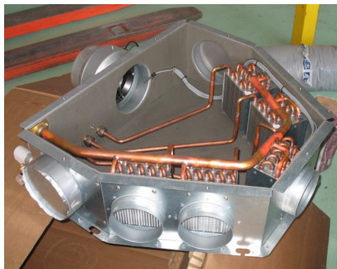
Figure 4 : Vue de côté de la dernière version du prototype, version 5 sorties d'air
