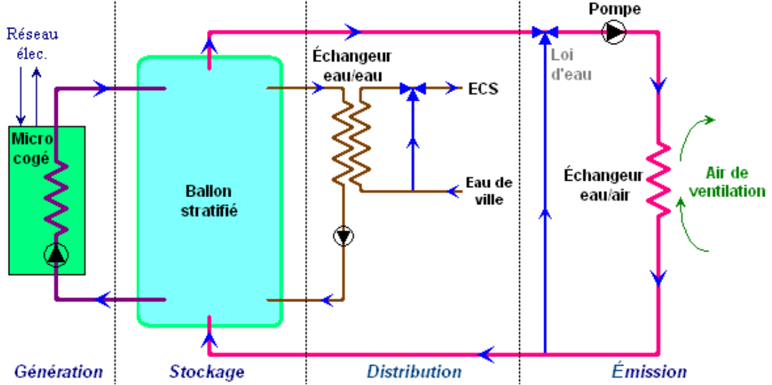
Figure 2 : Schéma général du système de chauffage et d'ECS étudié
