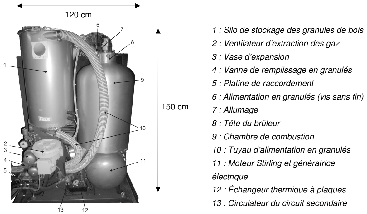
Figure 1 : Vue de l'unité de micro-cogénération à bois étudiée.
