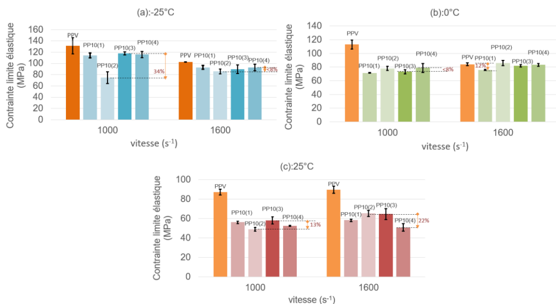
Fig. 11. Comparaison entre les lots différents lot de PP10 recyclés, Contrainte à la limite élastique : (a) -25°C, (b) 0°C, (c) 25°C.
