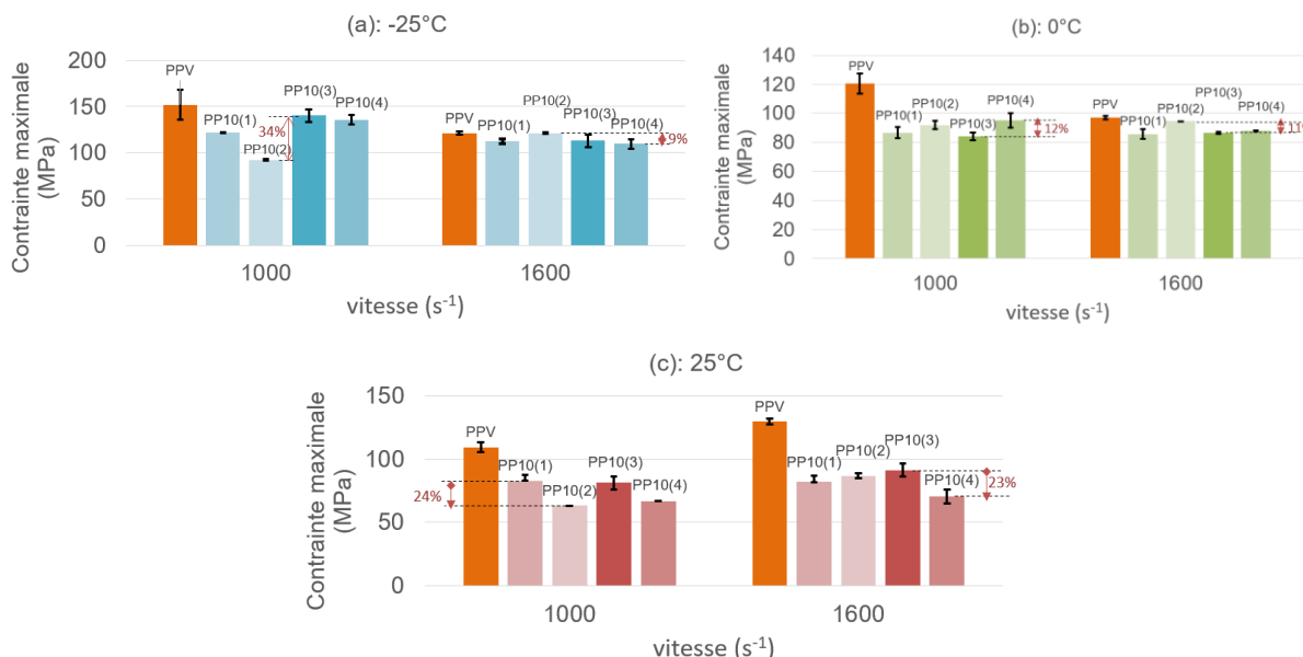
Fig. 12. Comparaison entre les lots différents lot de PP10 recyclés, Contrainte maximale : (a) -25°C, (b) 0°C, (c) 25°C.
