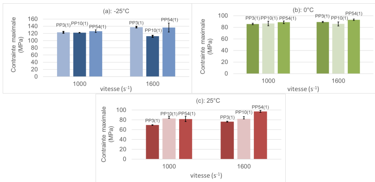
Fig. 5. Impact des grades, des additifs et/ou des contaminants sur la contrainte maximale en compression dynamique, (a) T1=-25°C, (b) T2=0°C, (c) T3=25°C.
