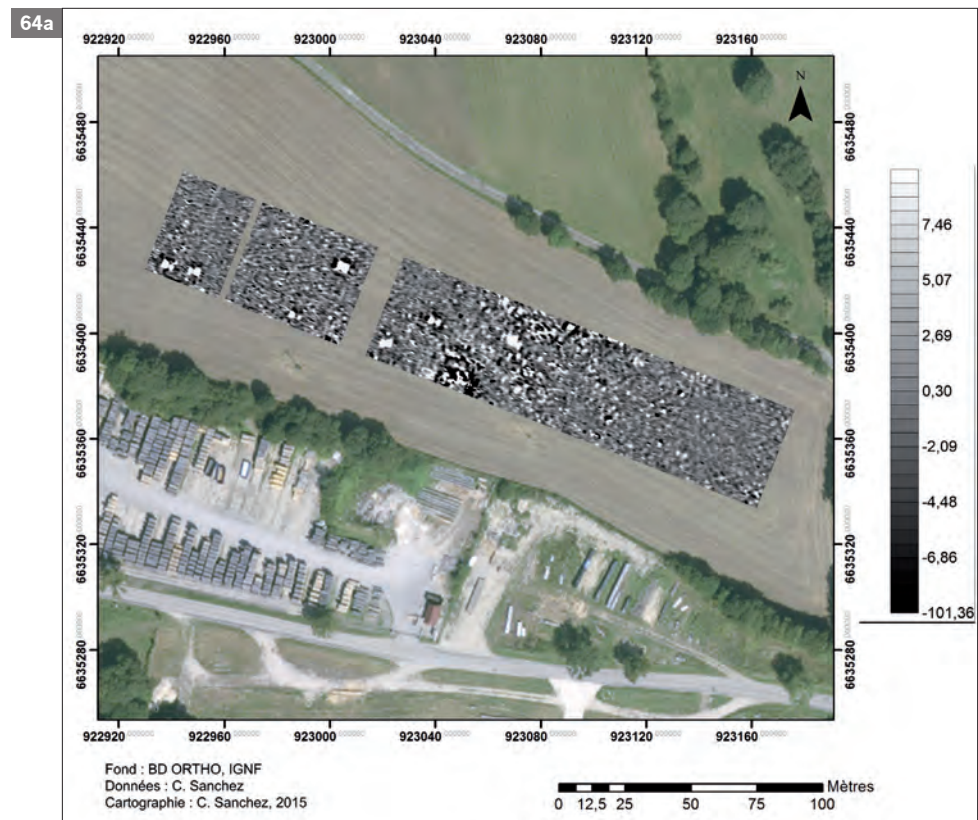
Fig. 64a, b et c Zone est, résultats des acquisitions de la prospection magnétique, Saint-Germain-en-Montagne (39).
