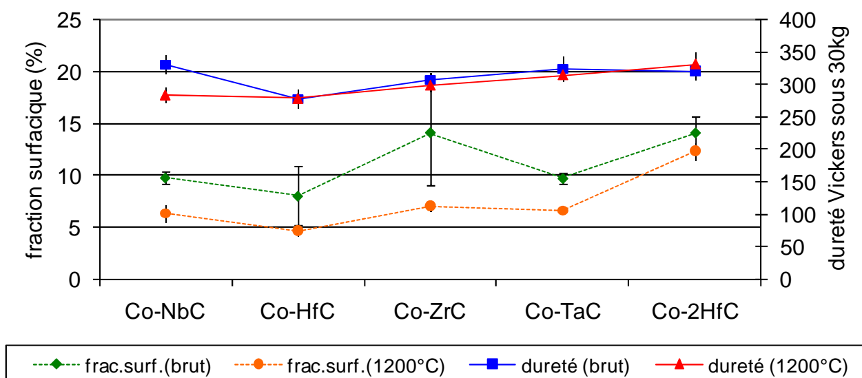
Figure 7. Fractions surfaciques de carbures et dureté Hv30kg
