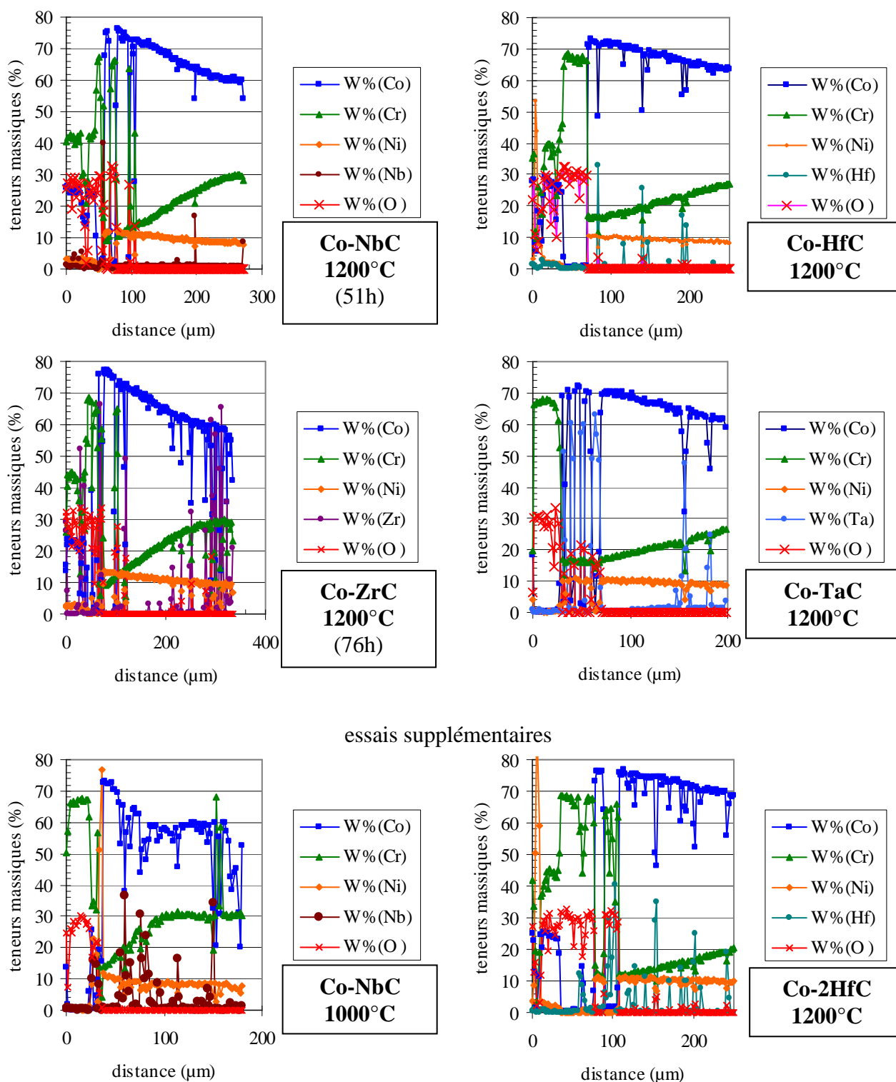
Figure 5. Exemples de profils de concentration réalisés au travers des couches d’oxydes superficielles et des zones d’alliage affectées par l’oxydation
