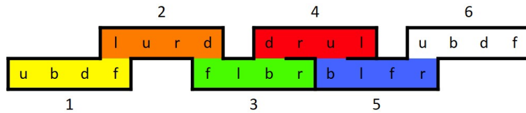
(d) Unfolded inner faces of a (1, 1, 1) -Menger polycube.
