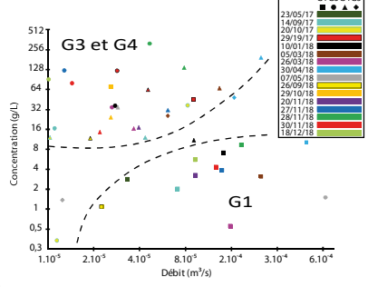
Figure 10. Diagramme des concentrations et débits des échantillons de matières en suspension
