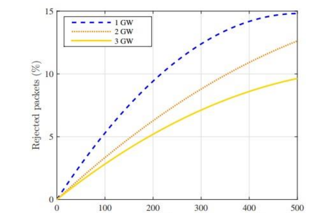
Fig 7.2 : Paquets rejetés en utilisant LoRa+ en fonction de nombre de passerelles
