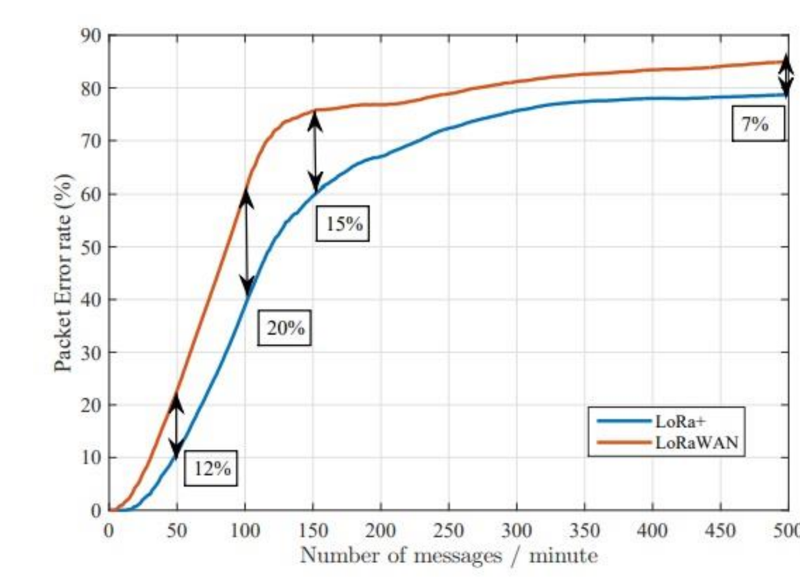
Fig 8: Paquets erronés (PER) pour les petites et moyennes villes en utilisant une passerelle
