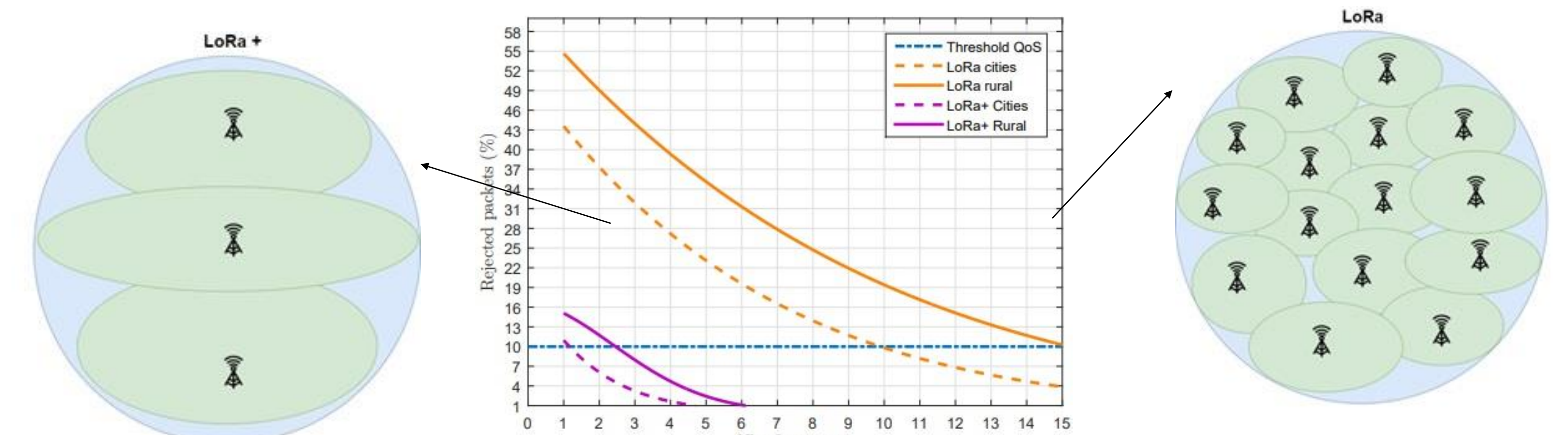
Fig 9: Comparaison du nombre des passerelles nécessaires entre LoRaWAN et LoRa+ pour une QoS définie
