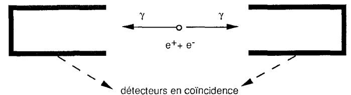
Figure 14a. – Détection de photons en coïncidence.
