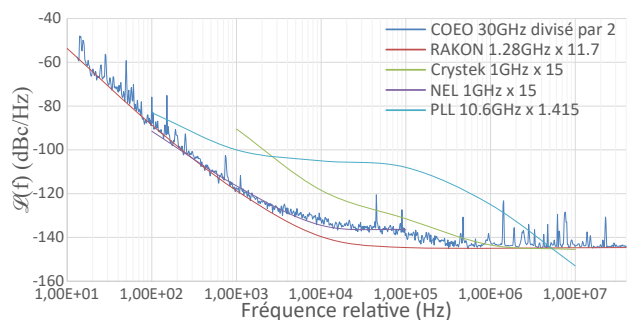
Figure 7. Bruit de phase du COEO divisé par 2 comparé à d'autres sources
