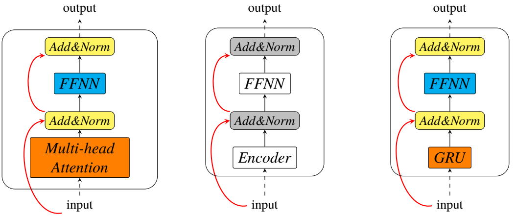
FIGURE 1 – Architecture générale, d’un point de vue conceptuel, de chaque bloc d’un réseau Transformer (au centre), sa réalisation pratique dans un modèle Transformer (à gauche) et sa réalisation dans notre réseau (à droite), dans lequel nous utilisons une couche GRU pour encoder des traits contextuels
