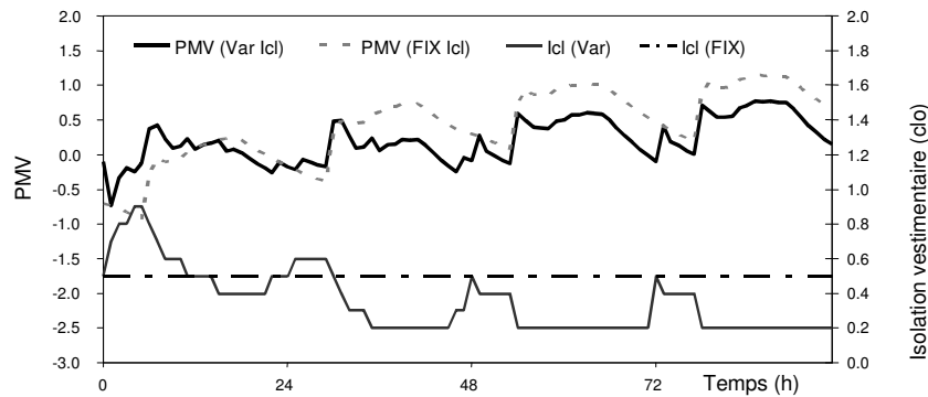
Figure 4: Variations du PMV avec habillage fixe (FIX) et habillage ajustable (Var) (bâtiment de forte inertie)
