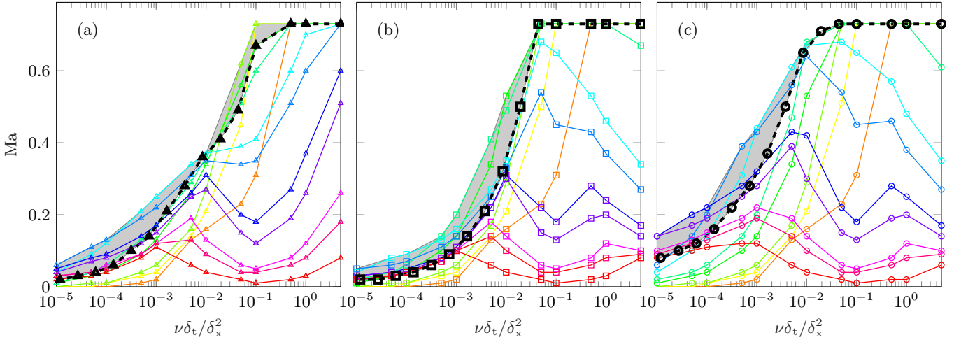
FIG. 2: Stability areas of the SRT (---) and LKS with EDFs of (a) second, (b) third and (c) fourth order, for different values of the free parameter: \eta\delta_t/\delta_x^2 = 5 (—), 1 (—), 5 \times 10^{-1} (—), 1 \times 10^{-1} (—), 5 \times 10^{-2} (—), 1 \times 10^{-2} (—), 5 \times 10^{-3} (—), 1 \times 10^{-3} (—), 5 \times 10^{-4} (—), 1 \times 10^{-4} (—), 5 \times 10^{-5} (—), 1 \times 10^{-5} (—).
