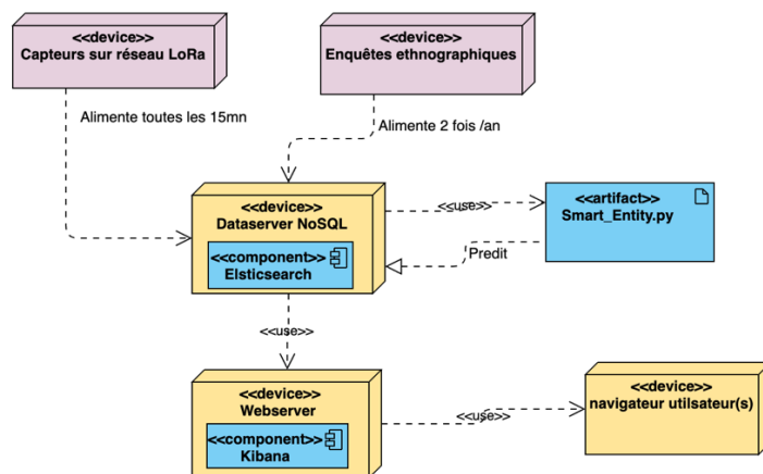
Figure 1 : Diagramme de déploiement simplifié du SIP du Smart Village
