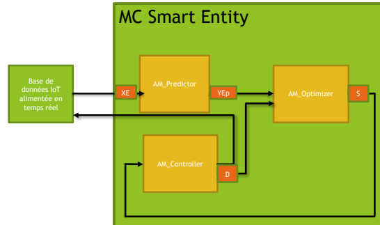
Figure 3 : le Modèle Smart Entity selon formalisme DEVS (Zeigler et al., 2000)
