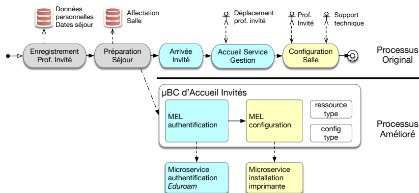
Figure 3 - Processus invité traditionnel versus processus amélioré par les µBC
