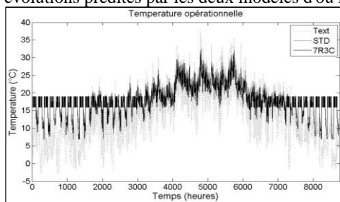
Figure 4 : Confrontation 7R3C - Pléiades sur année type - Suivi Température
