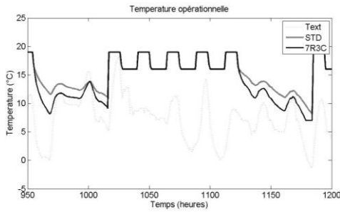
Figure 6 : Confrontation 7R3C - Pléiades sur semaine type - Suivi Température
