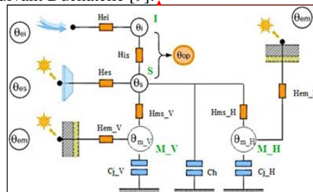
Figure 3-2: Le modèle 7R3C
