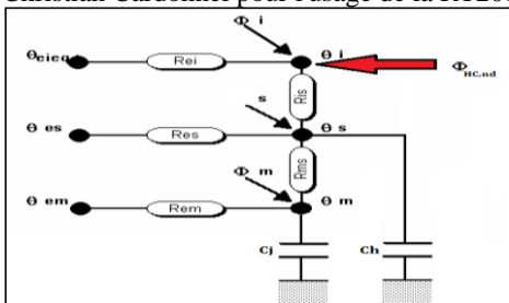
Figure 2-1: Le modèle 5R2C
