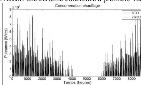
Figure 5 : Confrontation 7R3C - Pléiades sur année type - Suivi consommation
