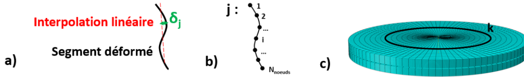
FIGURE 7 – a) Distance " \delta_j " entre le segment déformé et sa régression linéaire ; b) Distribution des nœuds le long du segment d'épaisseur " j ", au rayon fixé " k "; c) rayon fixé " k ", sur la plaque supérieure.
