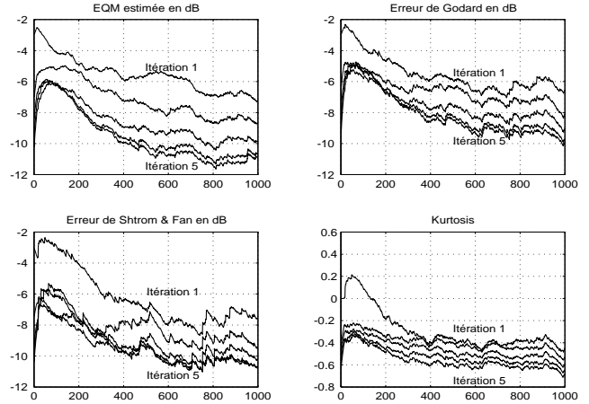
FIG. 5 : Signaux d'erreurs élaborés en ligne (EQM estimée, Godard, Strom & Fan et kurtosis).
