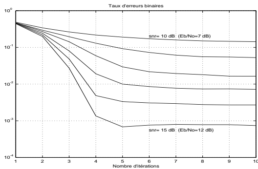
Fig. 4 : Taux d'erreurs binaires au fil des itérations.
