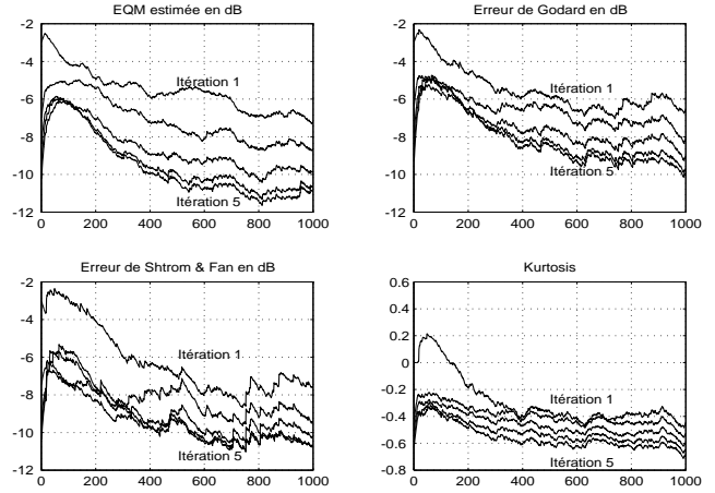
FIG. 5 : Signaux d'erreurs élaborés en ligne (EQM estimée, Godard, Strom & Fan et kurtosis).
