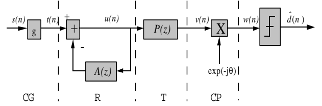
FIG. 1 : Egaliseur linéaire récursif
