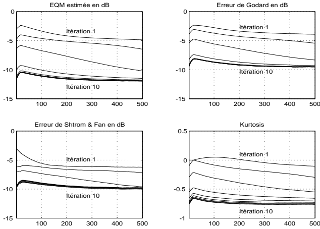
FIG. 3 : Signaux d'erreurs élaborés en ligne (EQM estimée, Godard, Strom & Fan et kurtosis), snr=15 dB.
