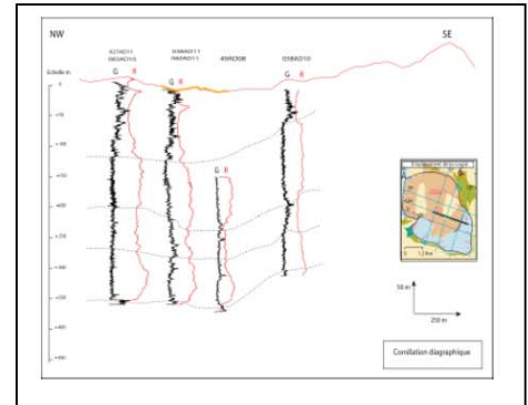
Figure 6 : Corrélation diagraphique
