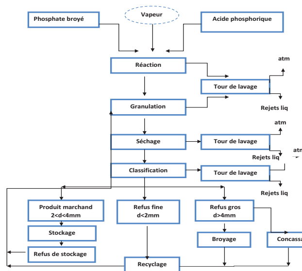
Figure1 : Schéma du procédé de fabrication TSP
