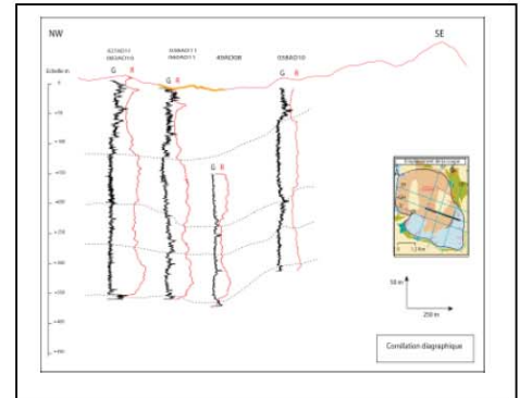
Figure 6 : Corrélation diagraphique
